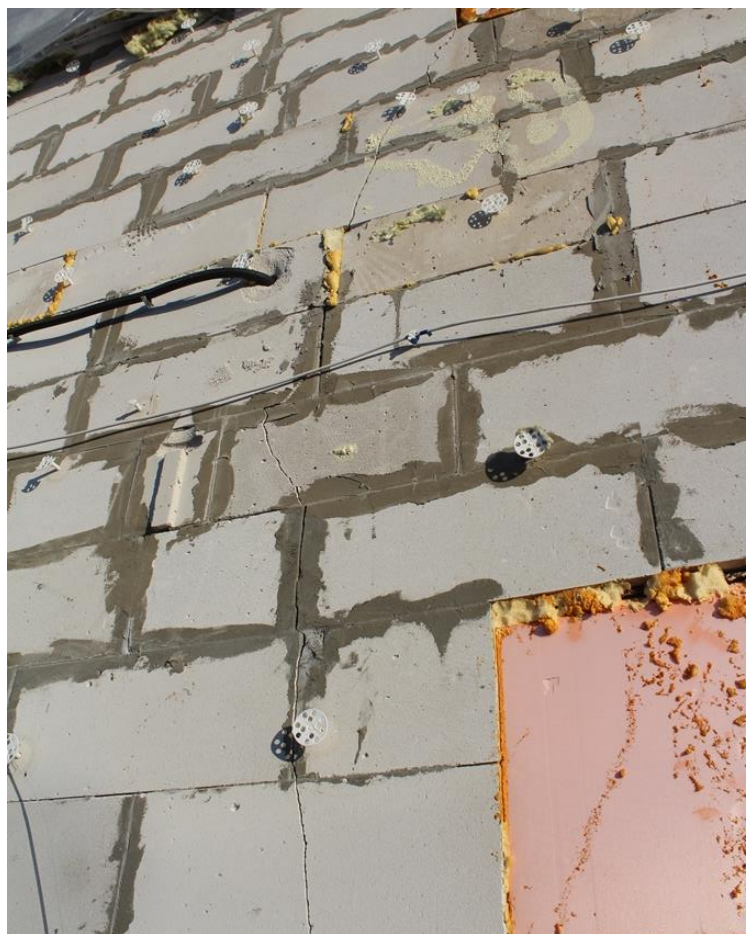
Фото 10. Трещина в кладке газобетонных блоков наружной стены
