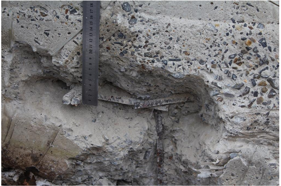
Фото 15. Замеры диаметра арматуры
