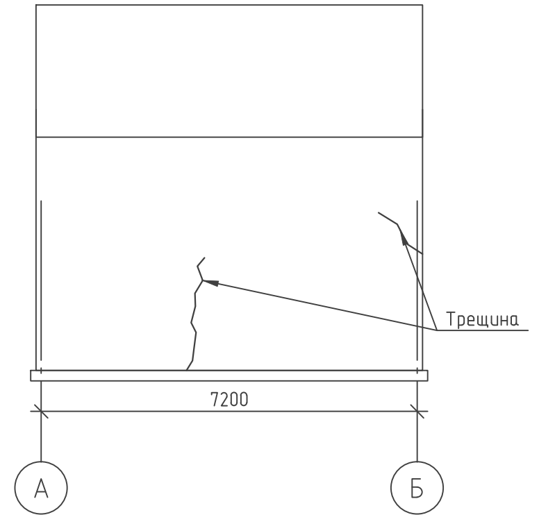
Фасад в осях 3;А-Б
