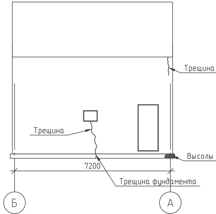
Фасад в осях 1;Б-А
